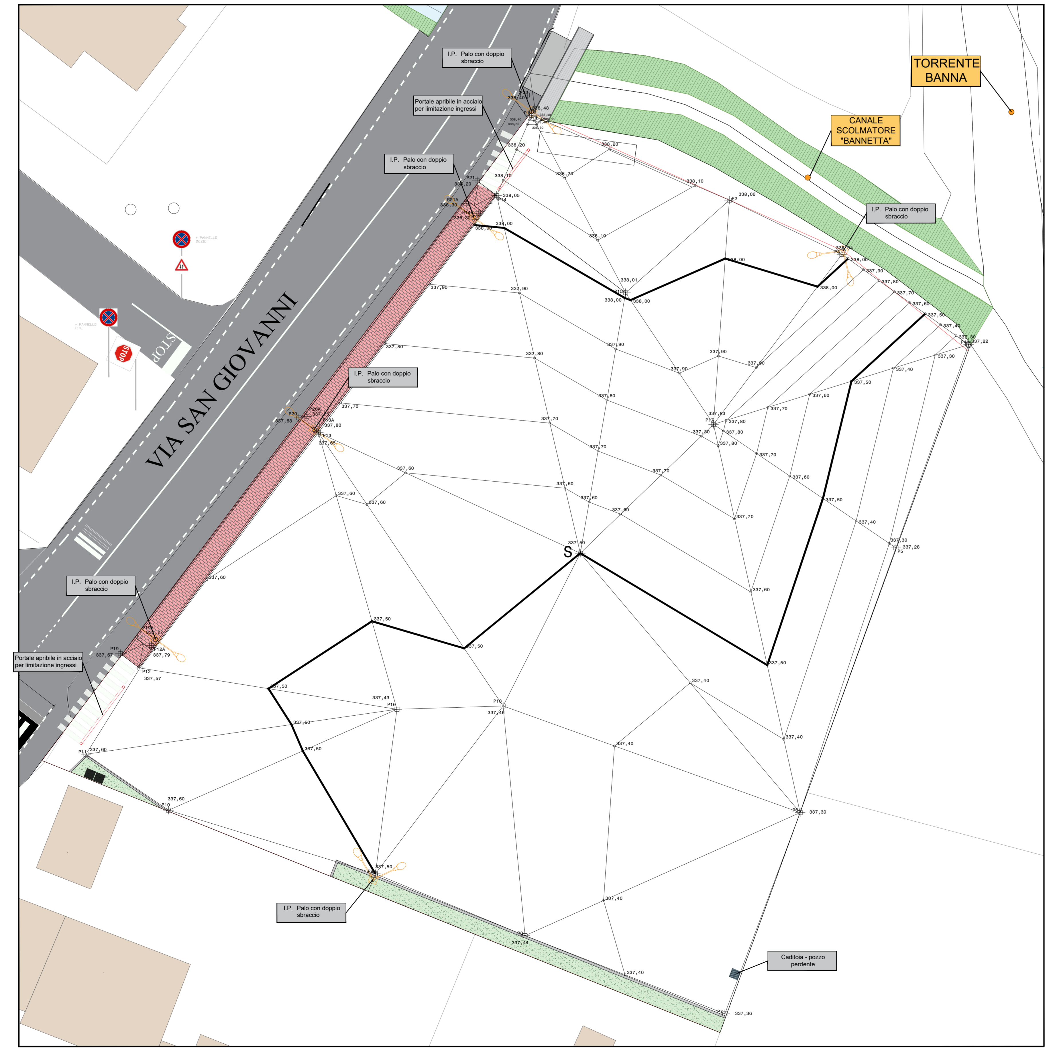
PLANIMETRIA AREA PARCHEGGIO GRANDE RILIEVO PLANO-ALTIMETRICO DELLE AREE E DEGLI SPAZI. COMUNE DI CIRIÉ - SCALA 1:200
