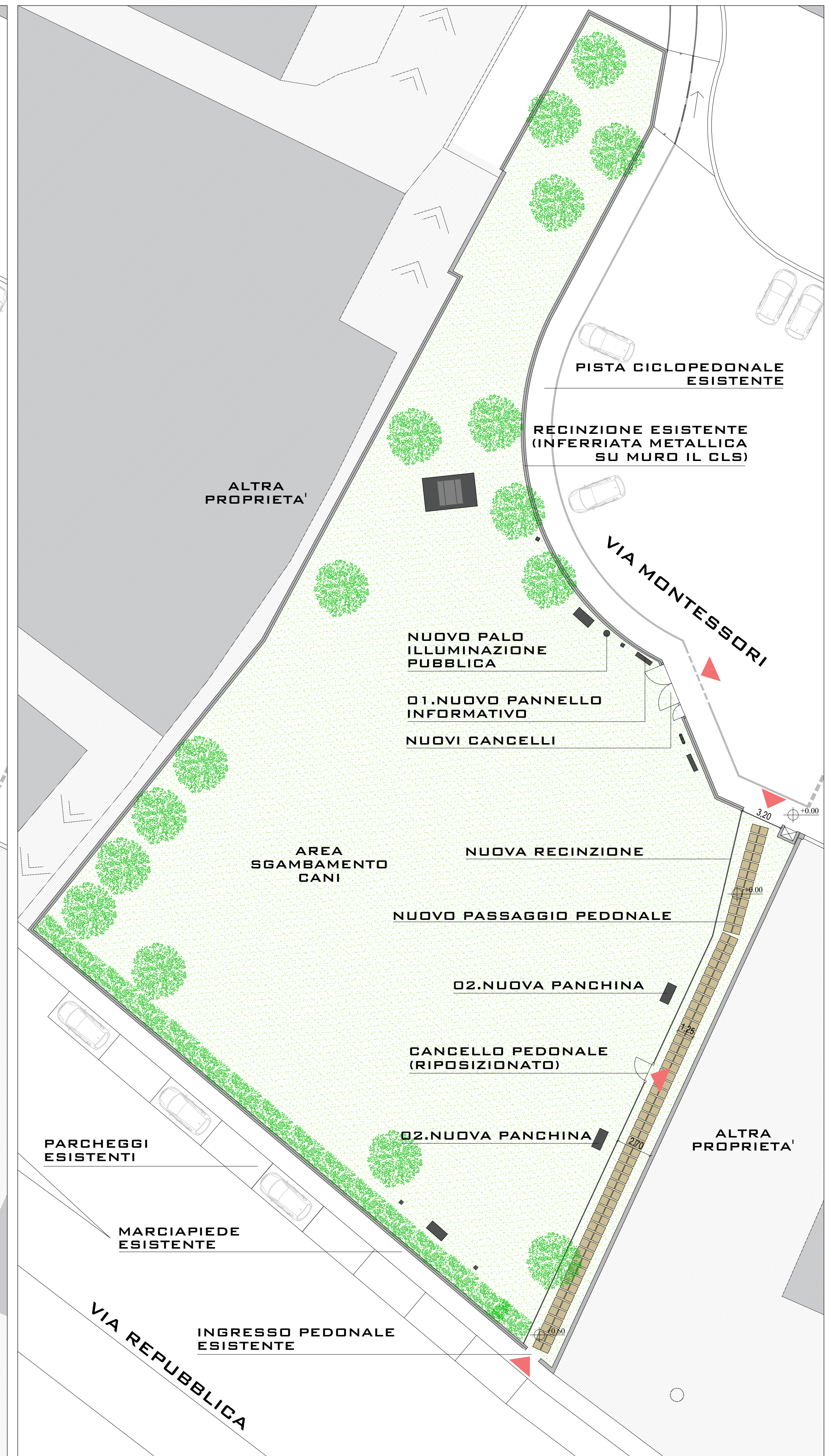
PLANIMETRIA DI PROGETTO
